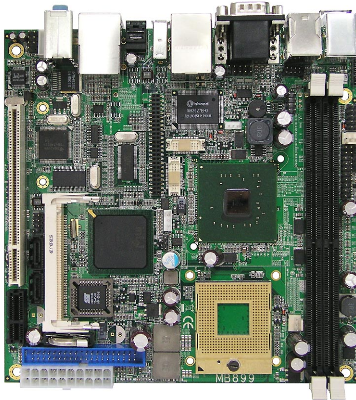
THE MB899 MINI ITX MOTHERBOARD
